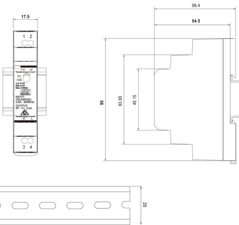
Fig. 2 Dimension bloc d'alimentation PSU2415
