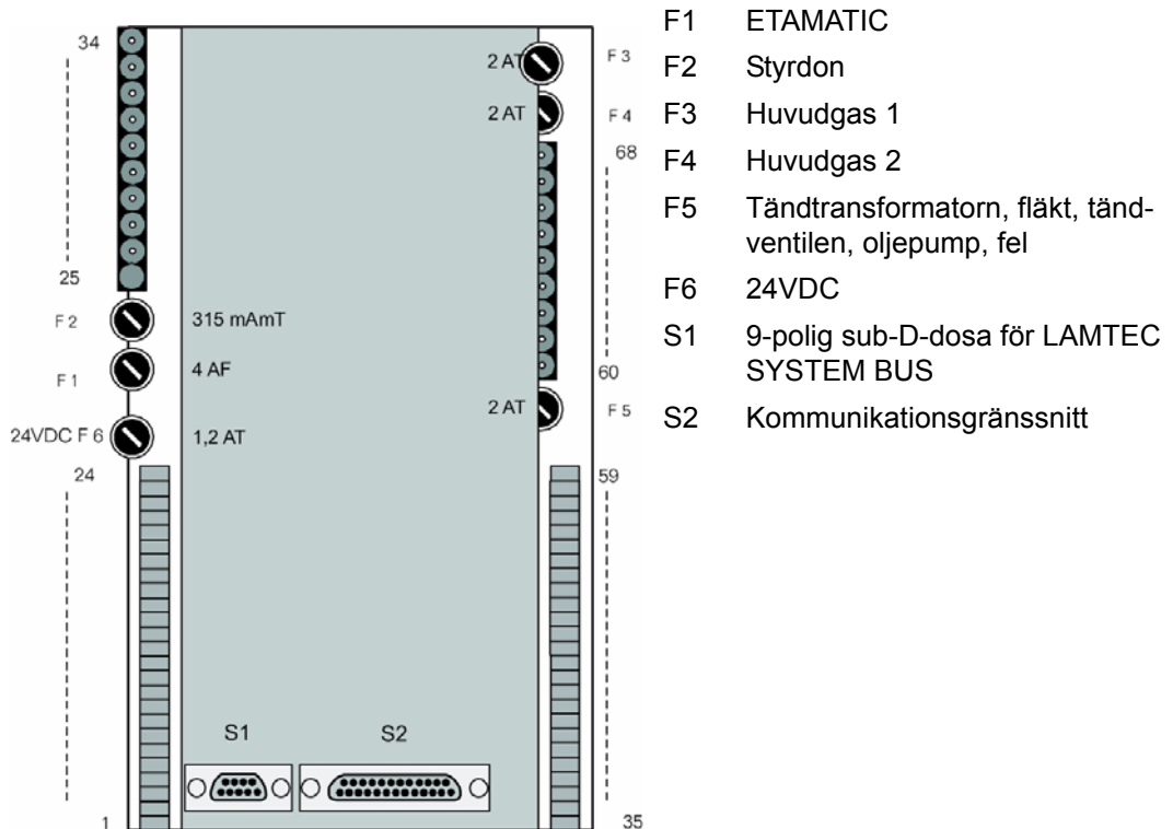
Fig. 8-11 Baksida ETAMATIC
