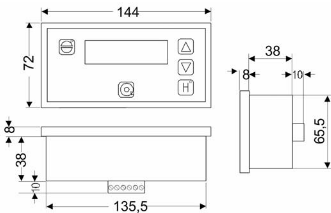
Fig. 8-7 Kundgränssnitt
