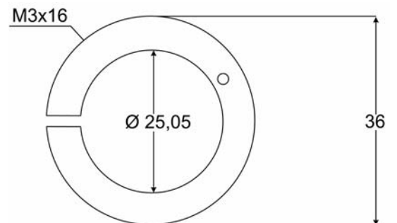
Fig. 8-15 Hållare för FFS 06, se även dokumentationen flamdetektor FFS 06 (DLT7502)
