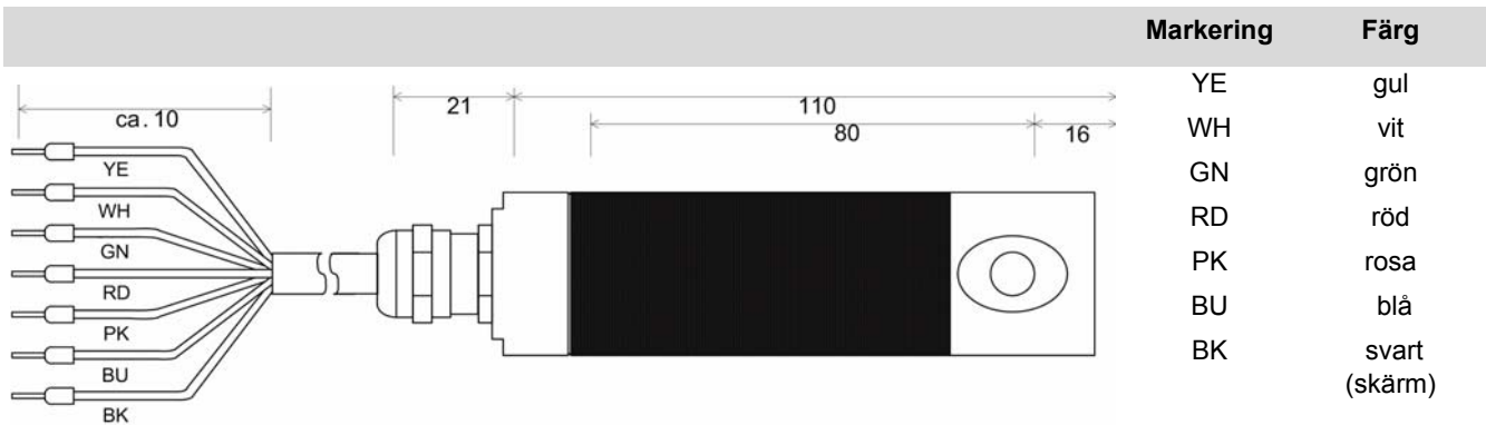
Fig. 8-12 Flamsensor FFS06 IR / VU
