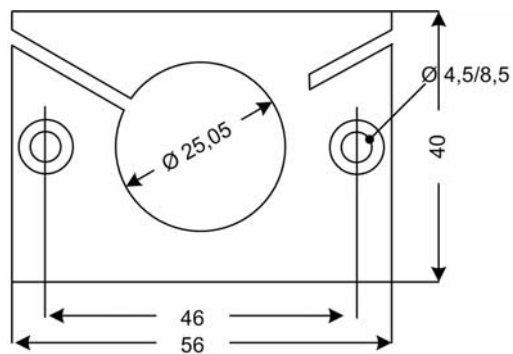
Fig. 8-14 Hållare FFS 05, se även dokumentationen flamdetektor FFS 05 (DLT7501 och DLT7503)
