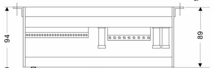
Fig. 8-10 Måttbild ETAMATIC
