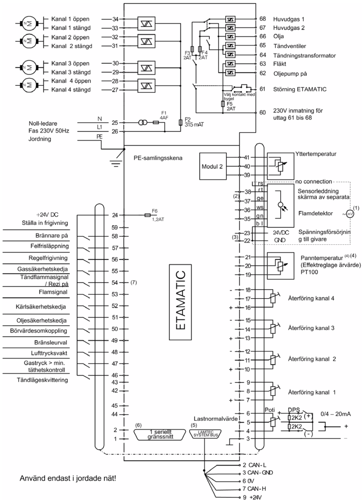
Fig. 8-5 Anslutningsbild ETAMATIC med tändflammebevakning
