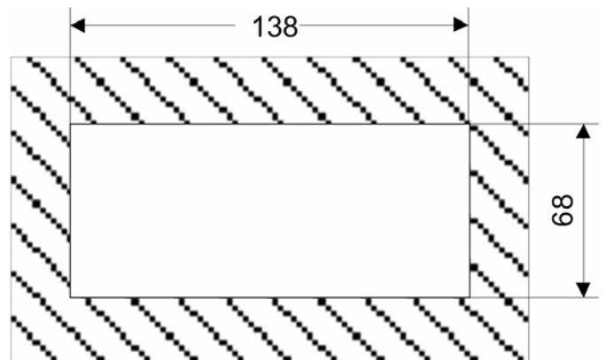
Fig. 8-8 Utsnitt ur kopplingstavla
