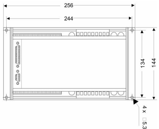
Fig. 8-8 Utsnitt ur kopplingstavla
