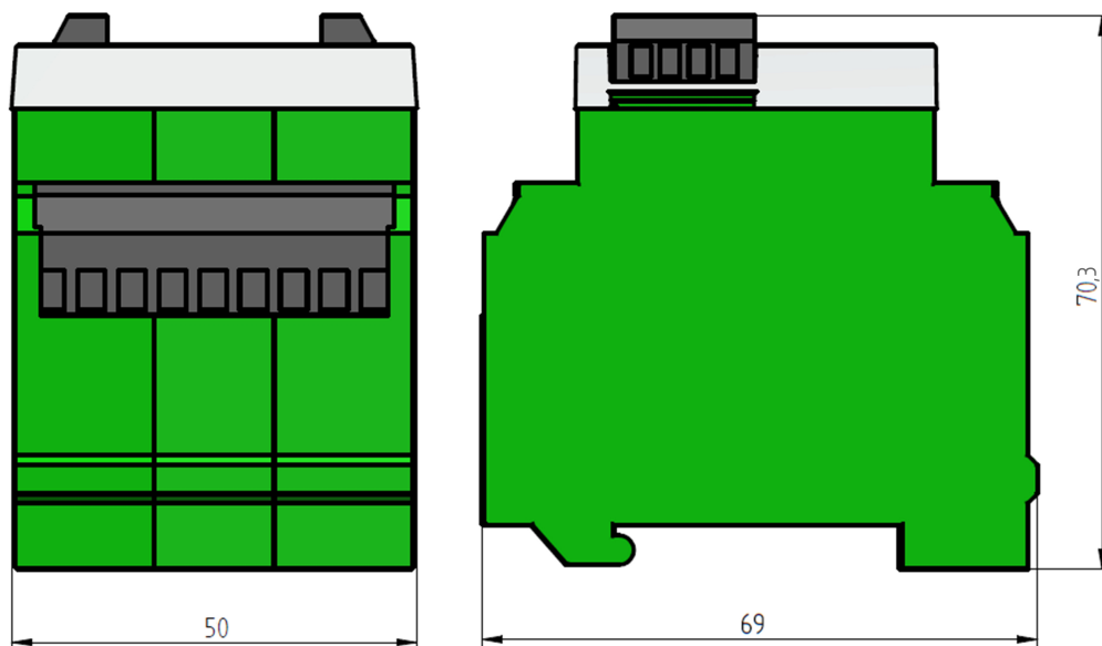
Fig. 1 Dimensions EBM100
